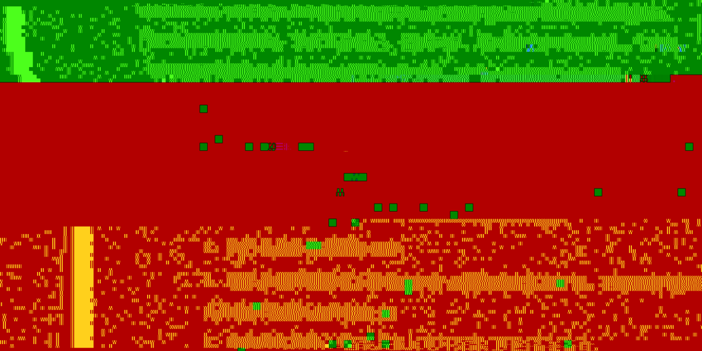
图 4-1 华新（丽江）环保新材有限责任公司石灰窑窑尾废气排口布袋除尘器除尘效率监测
